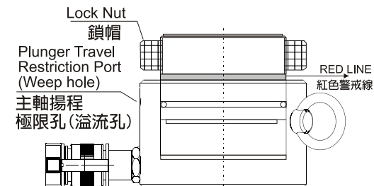
Plunger show at maximum extension 主軸全揚程示意圖
