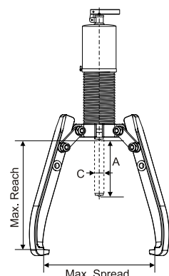
延長桿 Extend plunger
